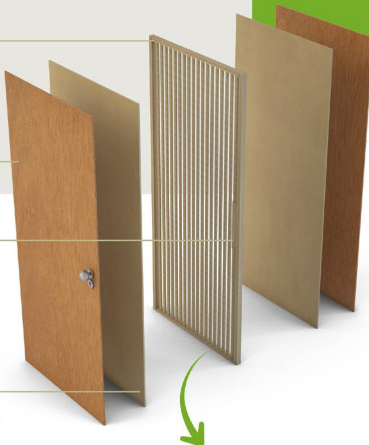
Contra-Capa em Chapa Dura ou em Lâmina de Pinus
